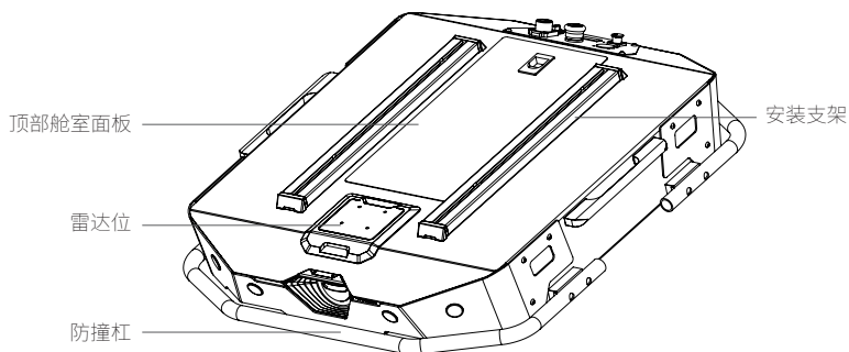
图2.1前部概览视图
