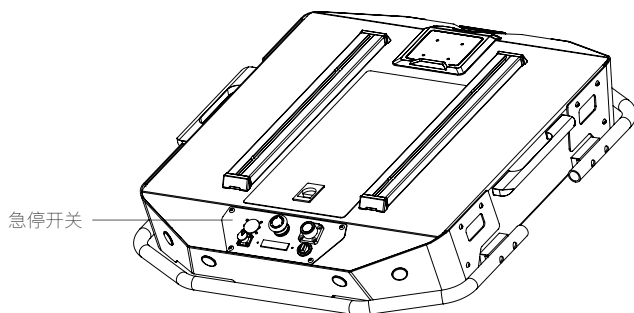
图2.2尾部概览视图
