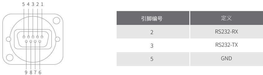
图 2.4 Q4 引脚说明图
